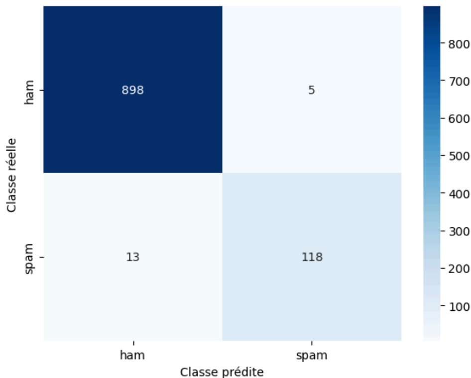
Matrice de confusion - Modèle 2 - DistilBERT
